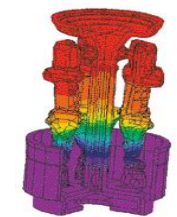
可以分析發生在晶粒選擇器中複雜的冶金過程
