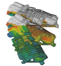
傾斜澆鑄鋁鑄件的充型過程視覺化
